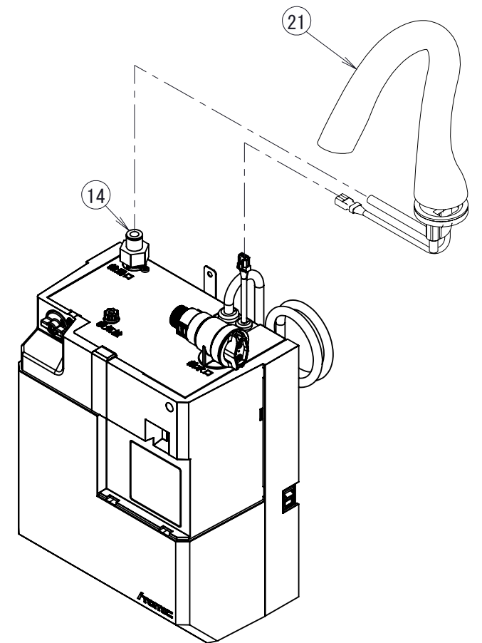
アイソメ図《自動水栓組立》
