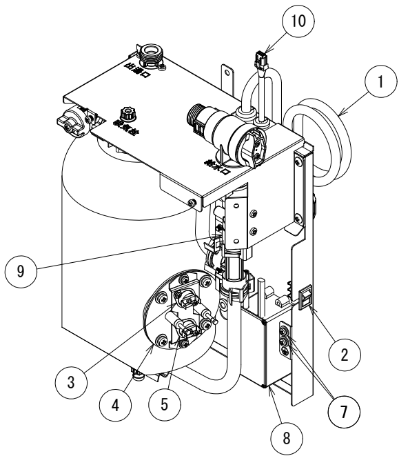
部品配置図 ESWM3ASW
