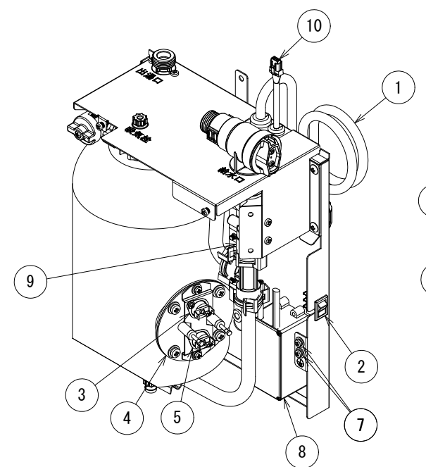
部品配置図 ESWM3ASK
