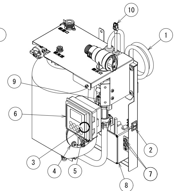
部品配置図 ESWM3TSK
