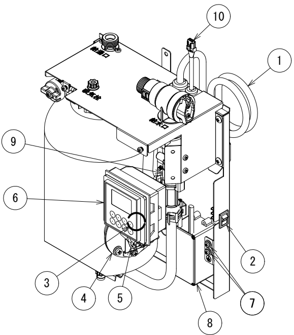
部品配置図 ESWM3TSK
