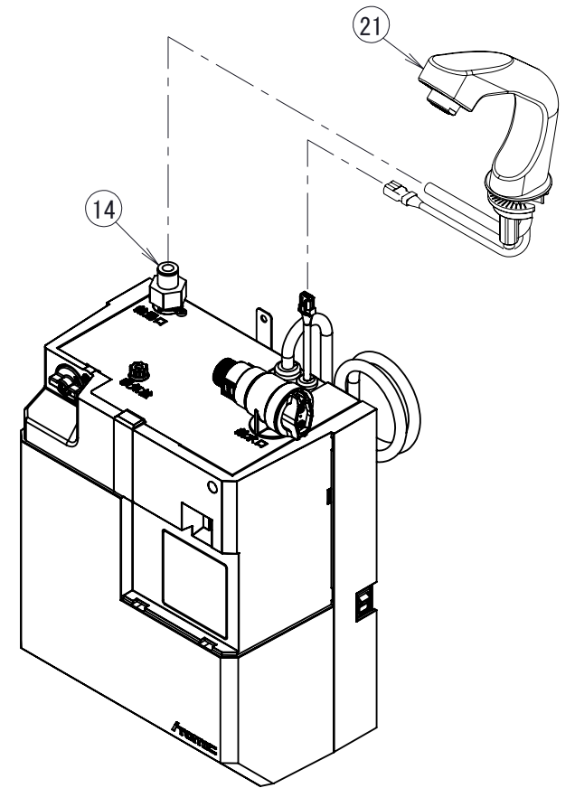
アイソメ図《自動水栓組立》
