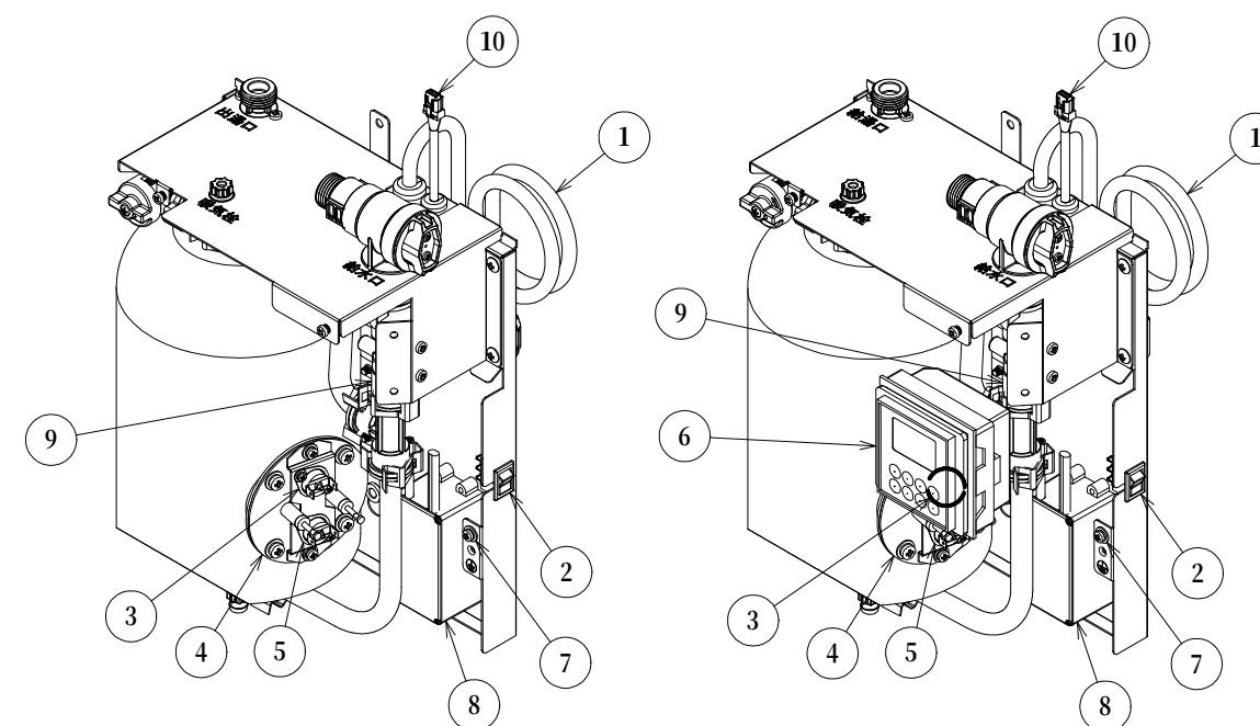
部品配置図 ESWM3ASS
