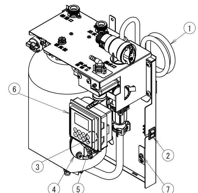
部品配置図 ESW03TTX
