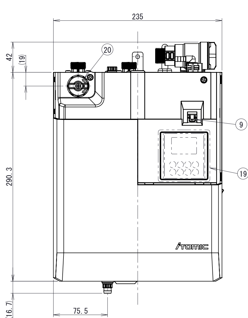
正面カバー取り外し状態詳細図
