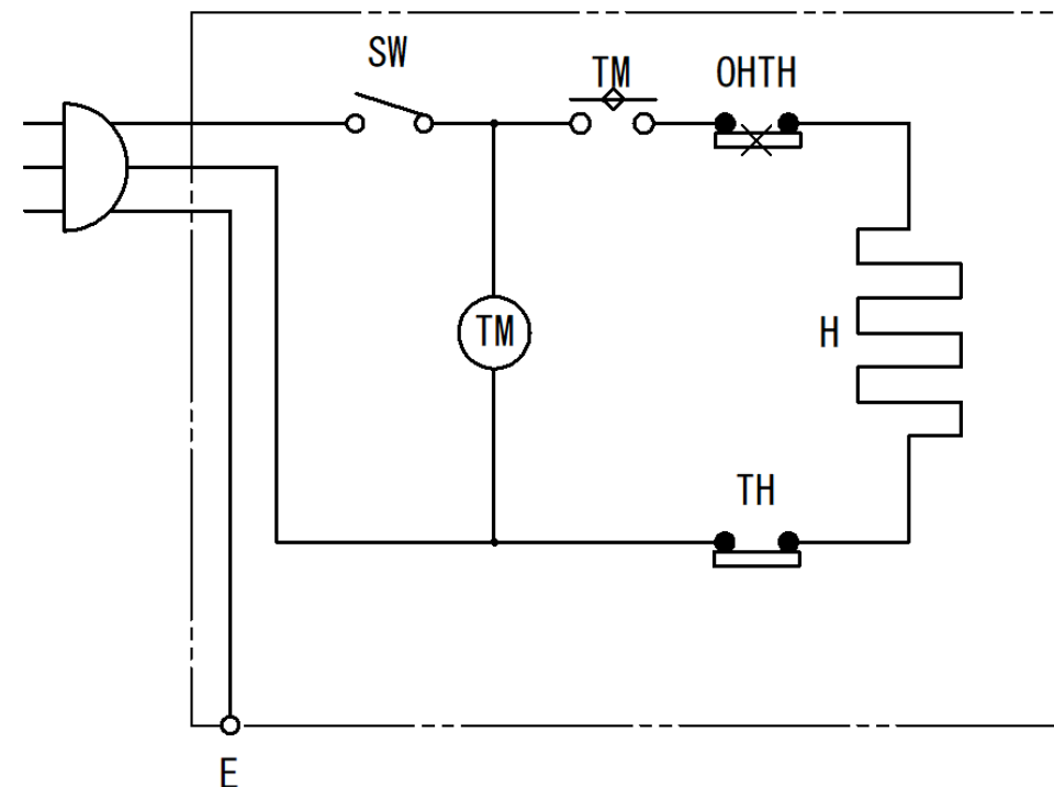
➡ ② ESW03TTX(デジタルタイマー付)
