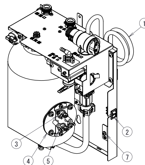
部品配置図 ESW03ATX
