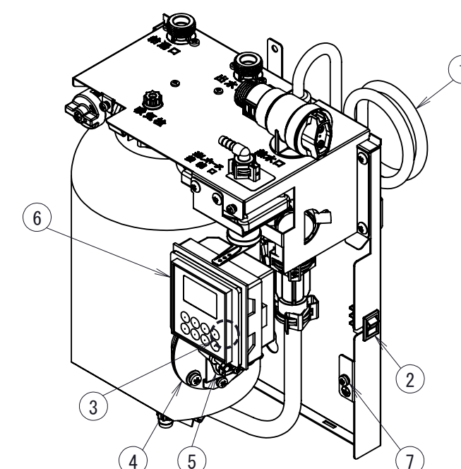
部品配置図 ESW03TTX
