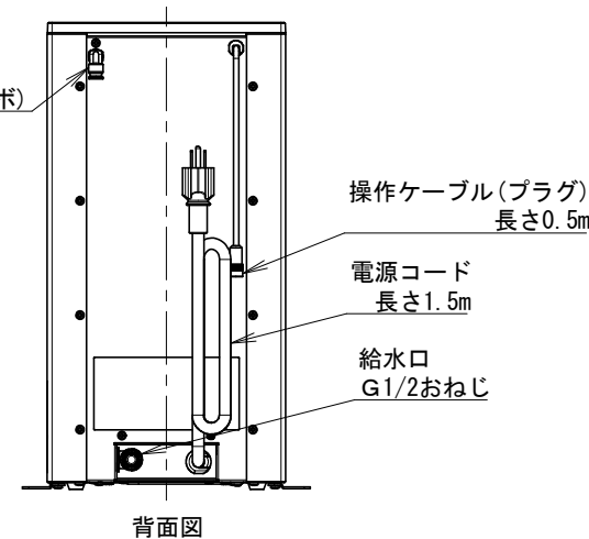
背面図
