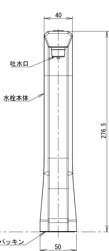
正面図
