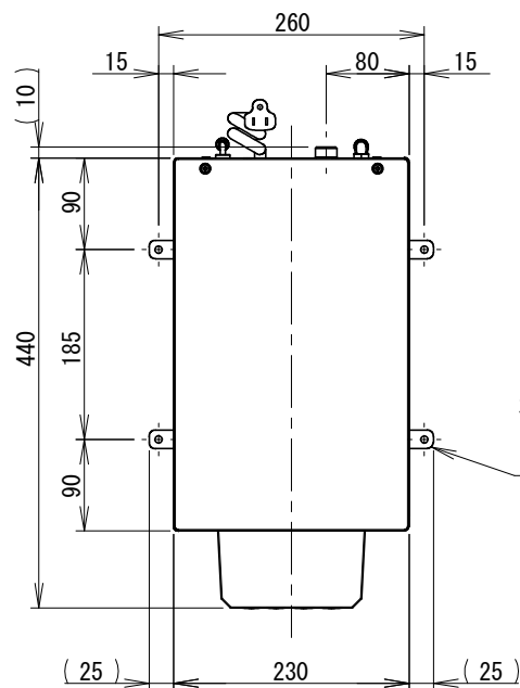
平面図
