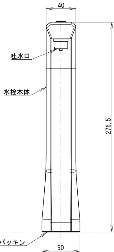
正面図
