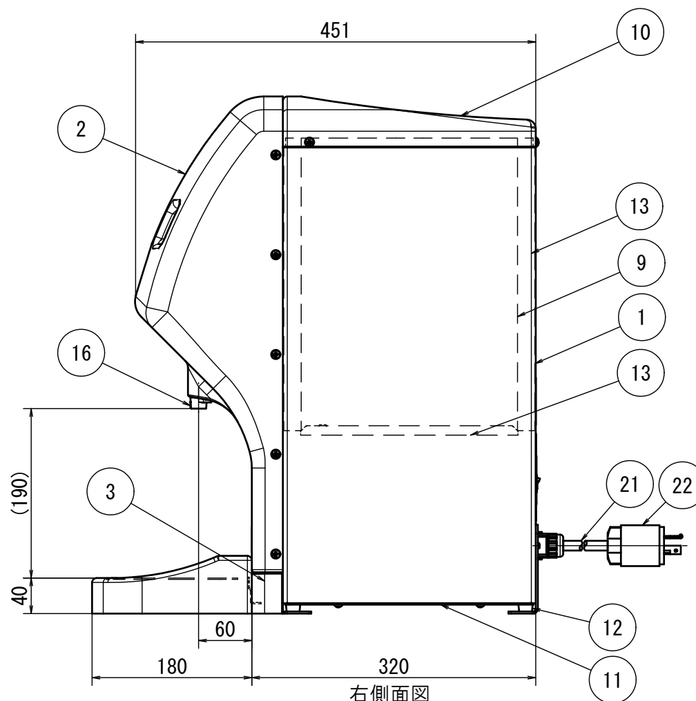
右側面図
