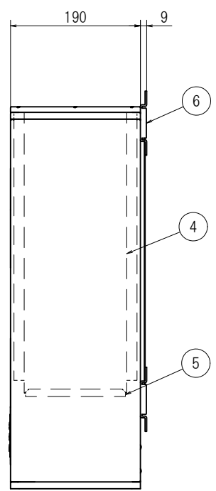
右側面図
