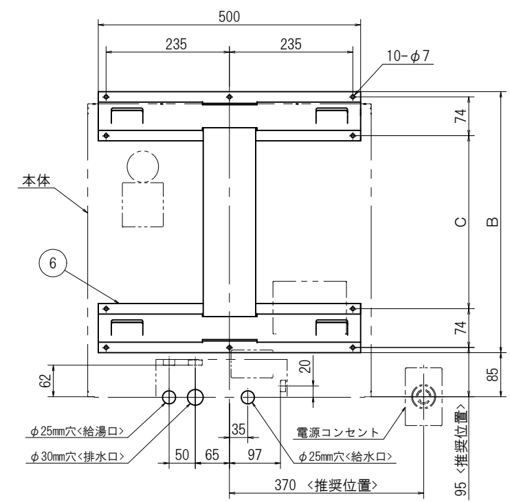
本体取付板寸法および取付例
