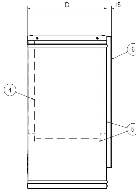
右側面図
