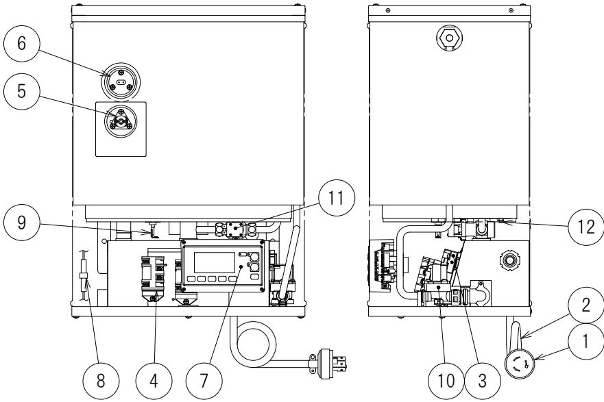
正面図
