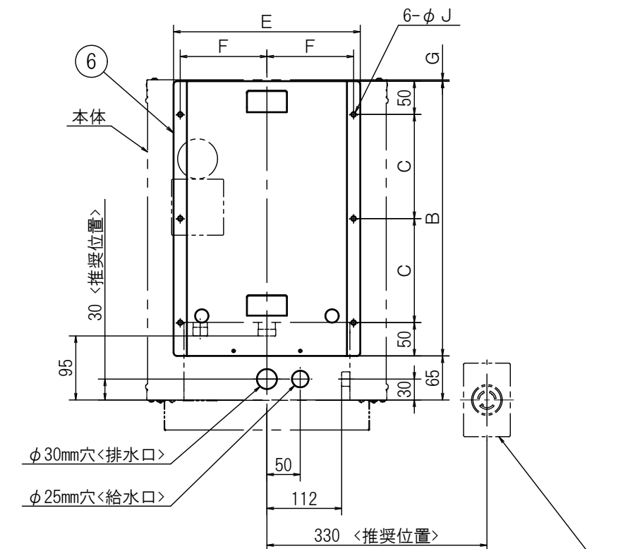
本体取付板寸法および取付例 電源コンセント
