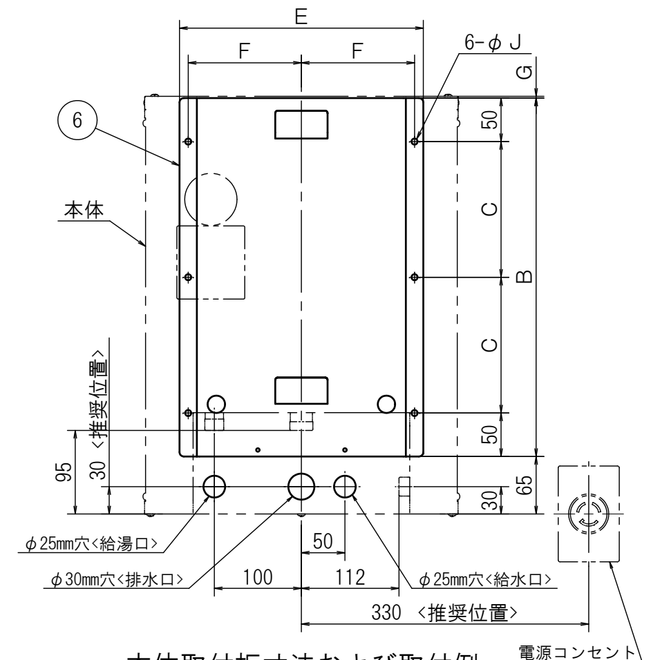
本体取付板寸法および取付例
