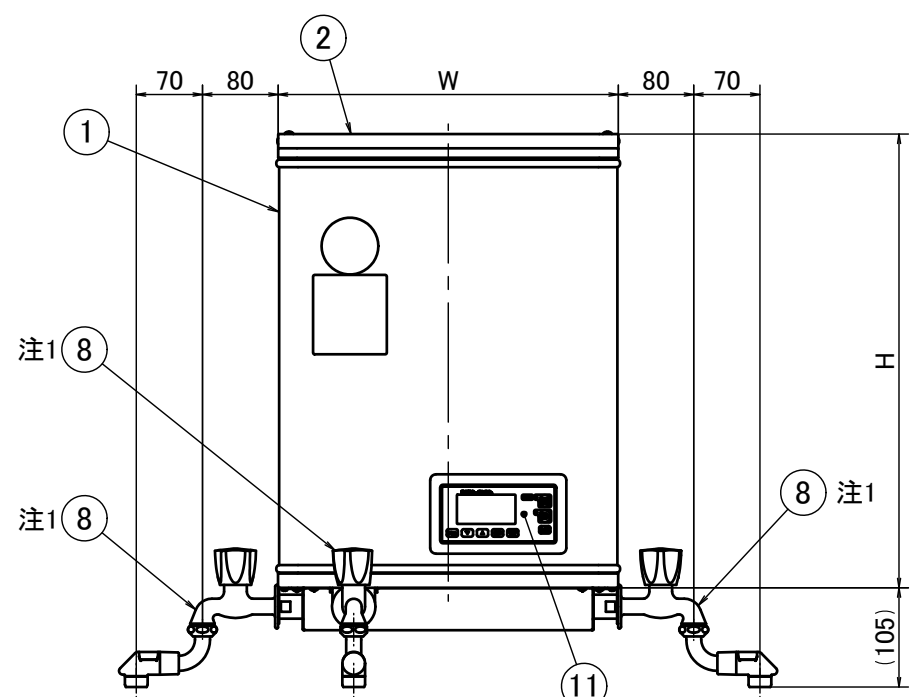
正面図
