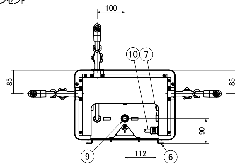
下面図
