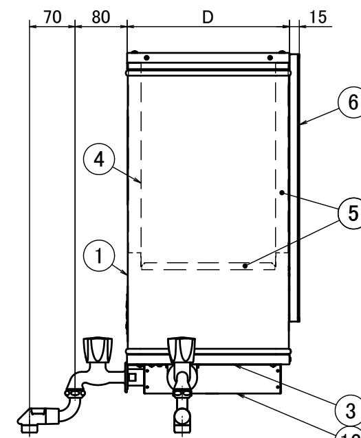
右側面図
