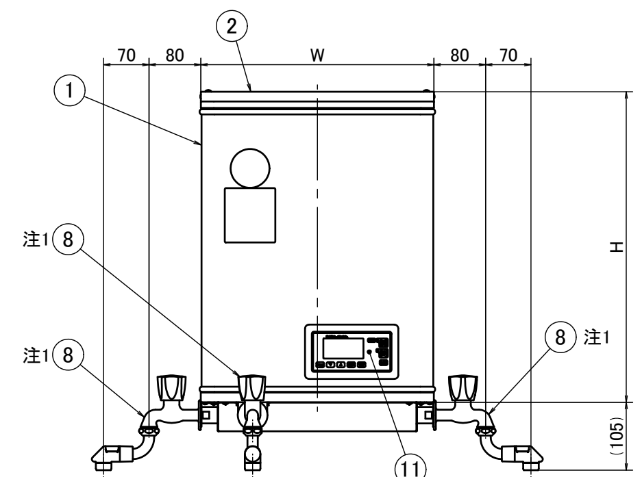
正面図
