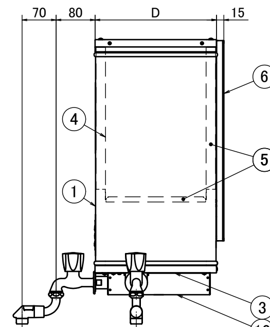
右側面図
