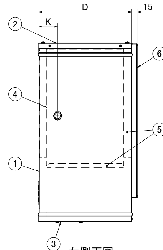
右側面図
