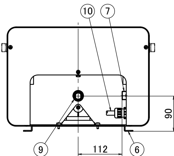
下面図
