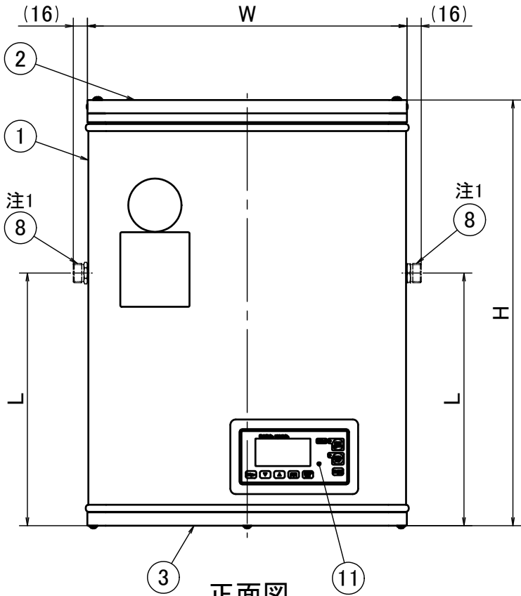
正面図
