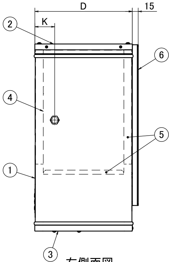
右側面図
