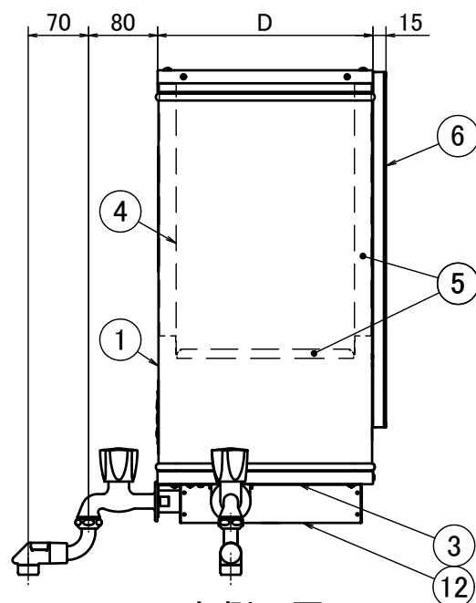
右側面図
