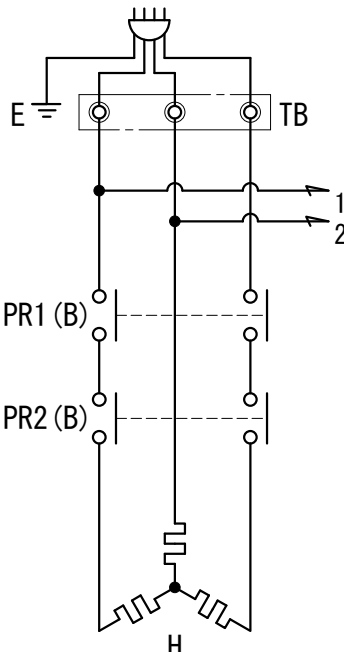
③ 三相
