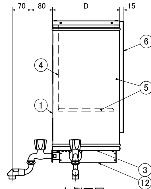
右側面図
