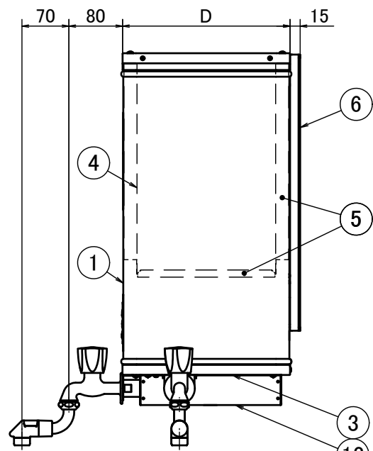
右側面図
