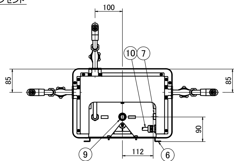
下面図
