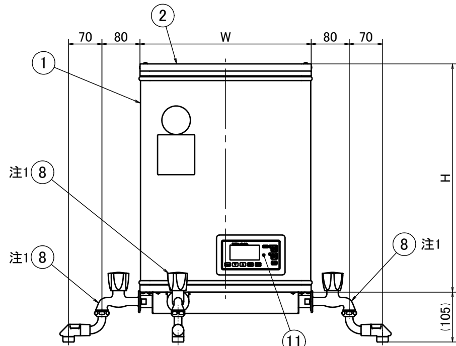
正面図
