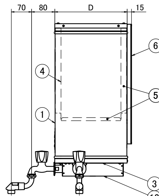
右側面図
