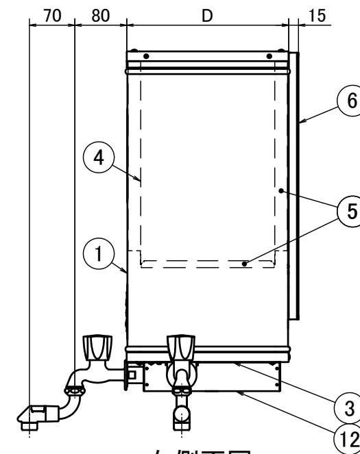
右側面図
