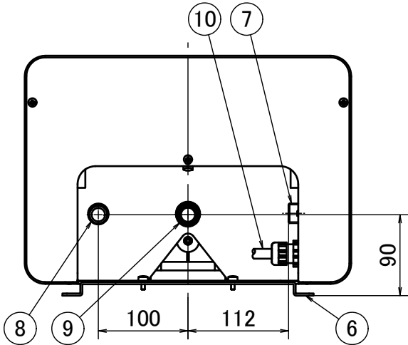
下面図
