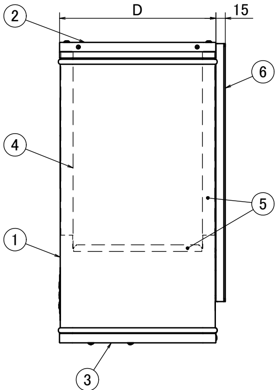
右側面図
