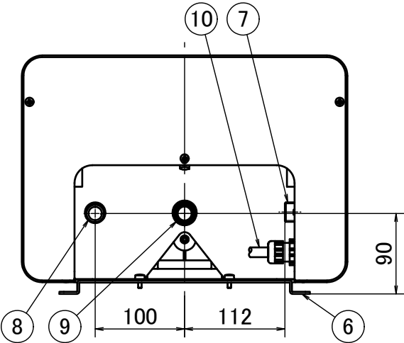
下面図
