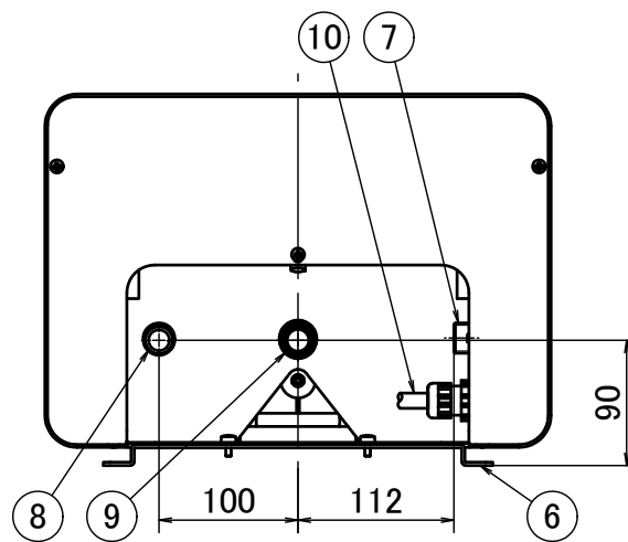
下面図
