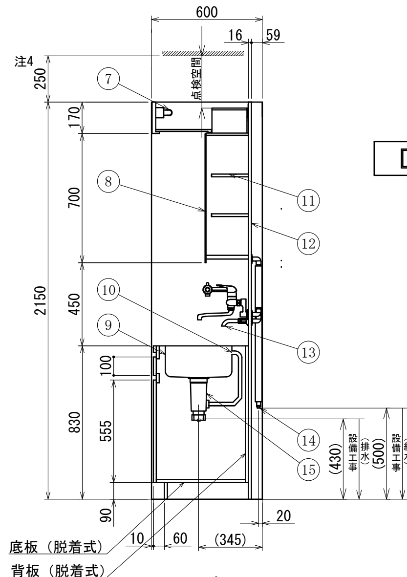
A-A'
