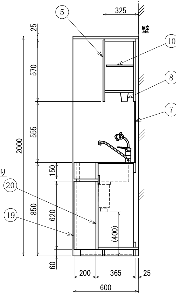
A - A'
