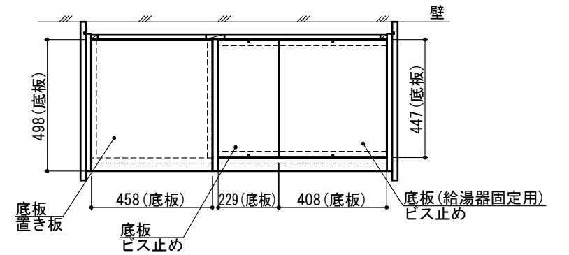
D-D' 断面
