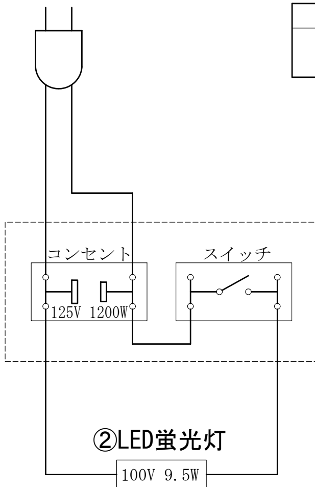
プラグ表
