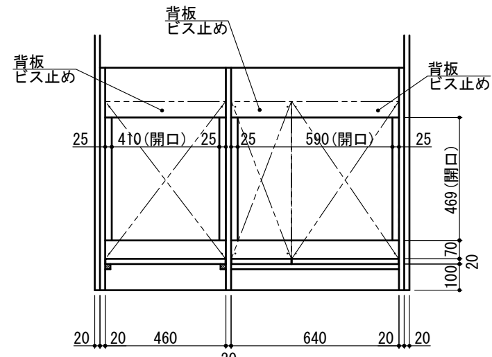
C-C' 断面
