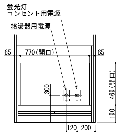
コンセント位置参考図 (背板を外した図)
