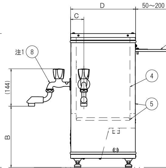
右側面図
