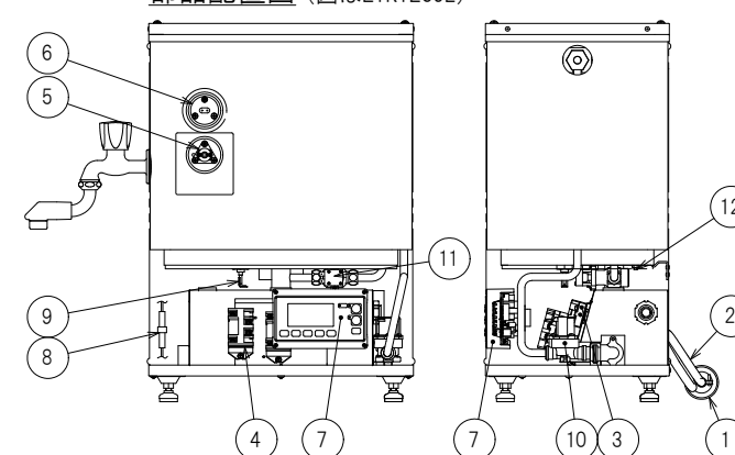
正面図
