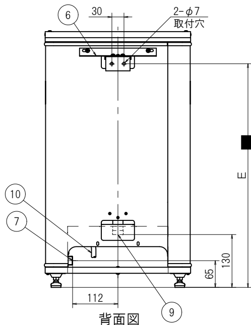
背面図
