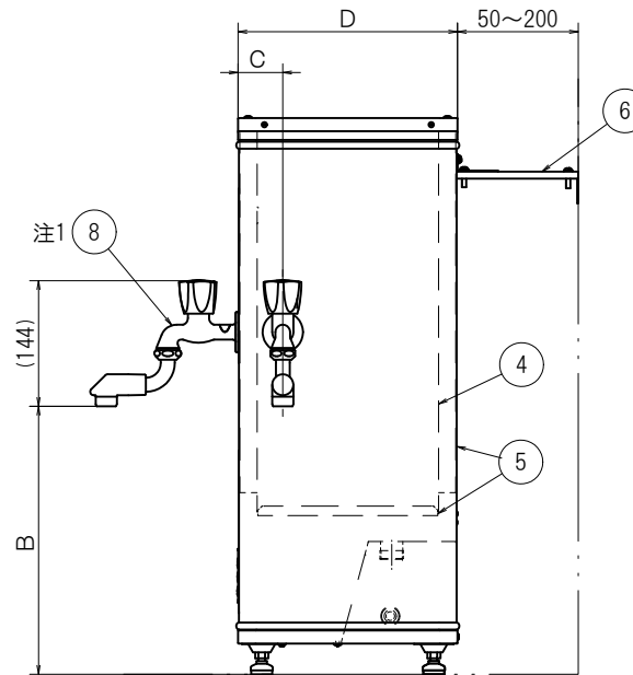
右側面図
