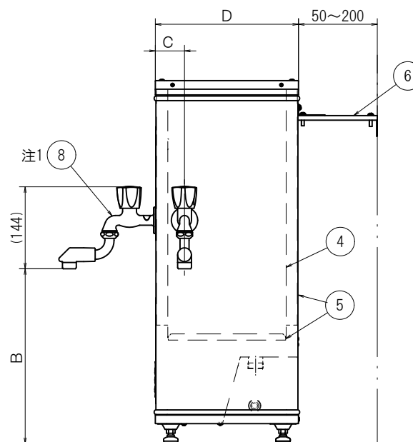
右側面図
