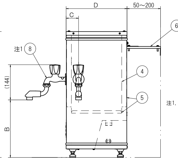
右側面図
