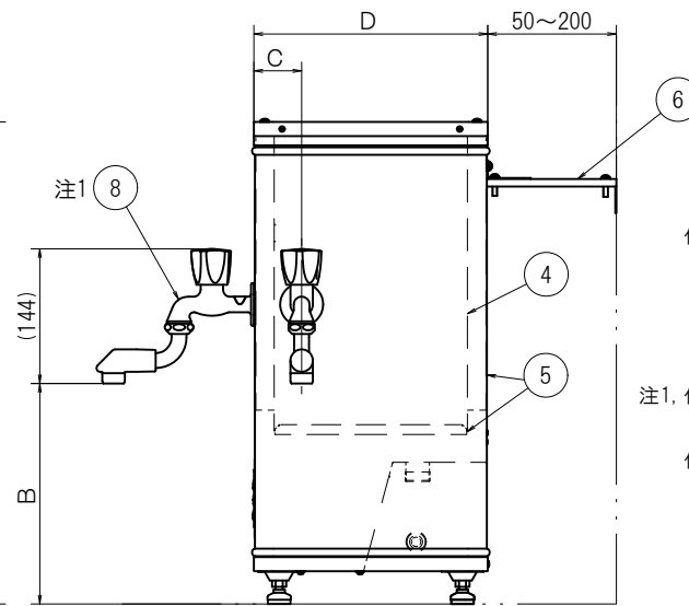
右側面図
