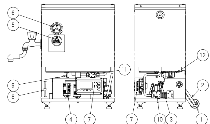
正面図
