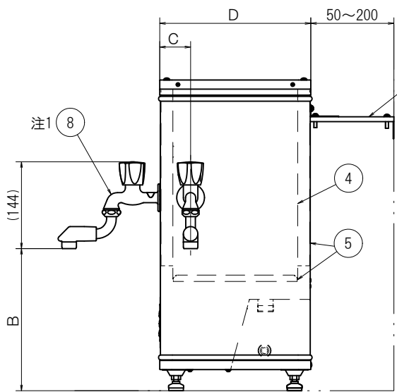
右側面図
