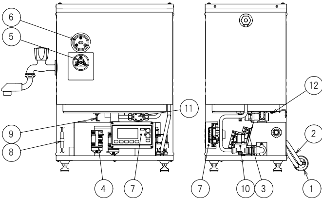
正面図
