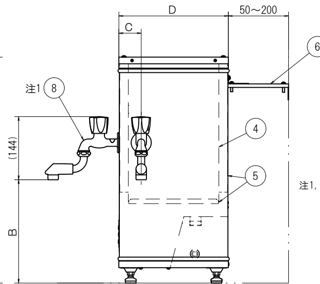
右側面図
