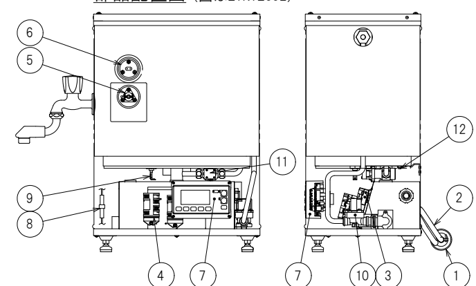
正面図
