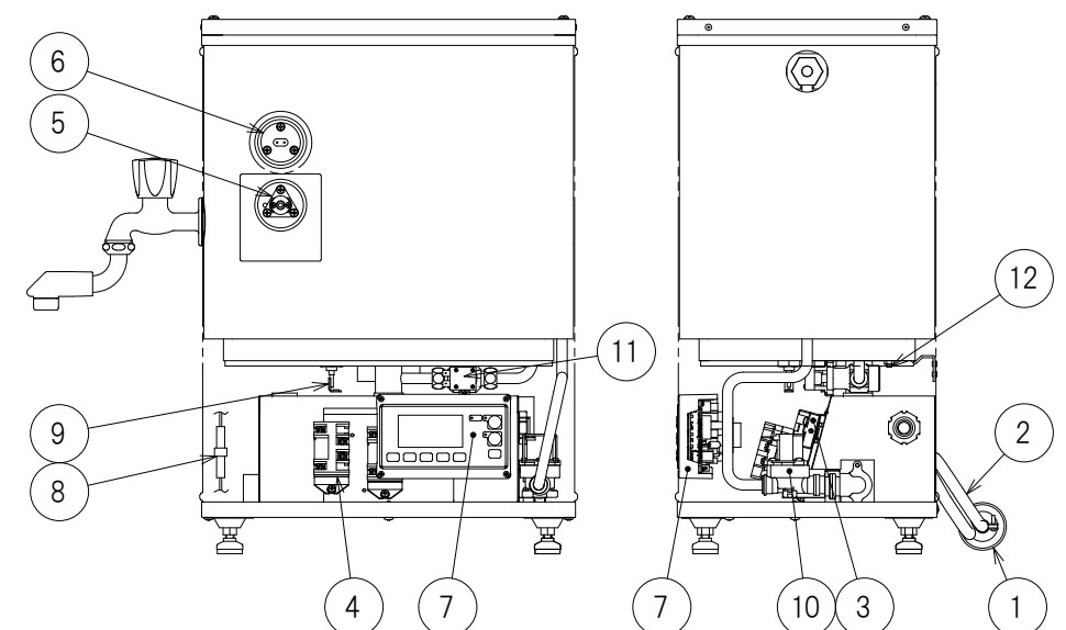
右側面図
