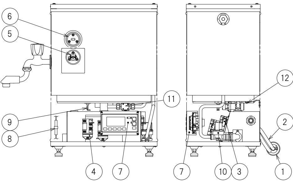
正面図
