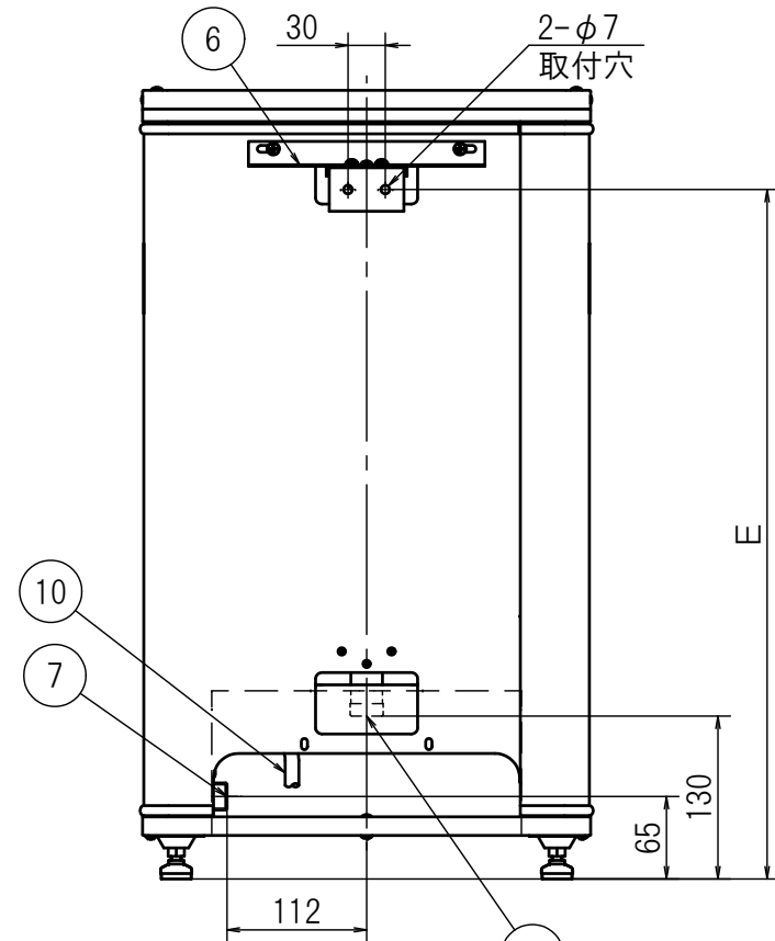
背面図
