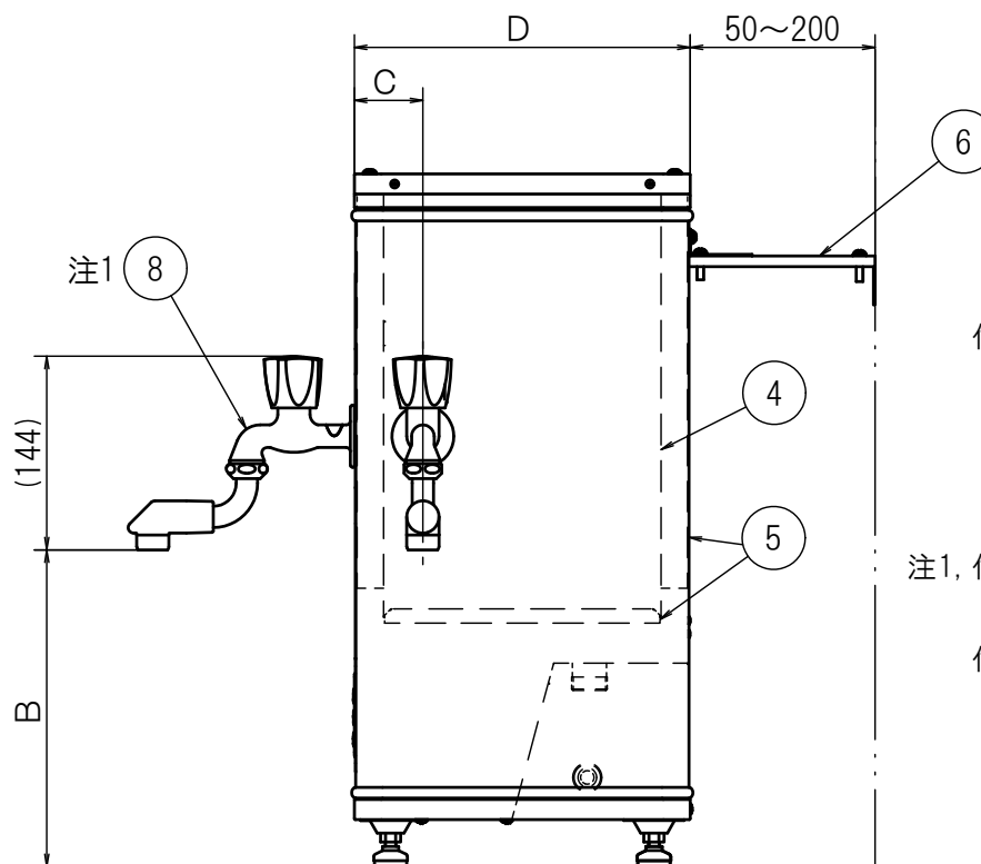
右側面図
